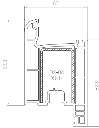
PRVN04 Kilitli Kapı Profili Door Sash Profile
