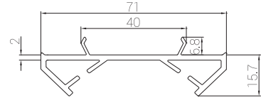
PR7127 Köşe Dönüş Adaptörü Corner Adapter
