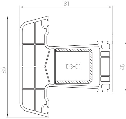
PRGR03 Orta Kayıt Profili Mullion Profile
