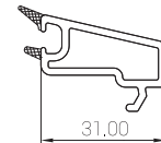
PRFS14 Tek Cam Çıtası Single Glazing Bead
