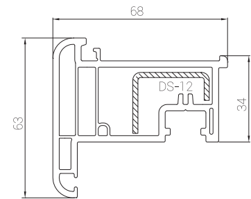
PR7113 Hareketli Orta Kayıt Profili Overhang (Stump)
