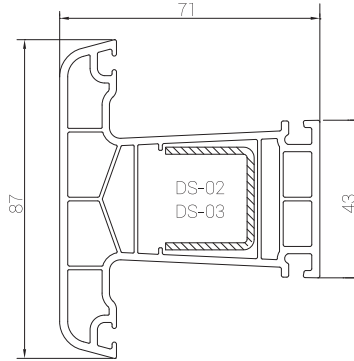
PRDR03 Orta Kayıt Profili Mullion Profile
