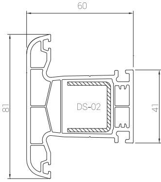
PRVN03 Orta Kayıt Profili Mullion Profile
