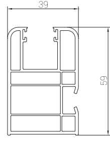
PRPJ91 59 mm Yan Dikme 59 mm Edge Pillar
