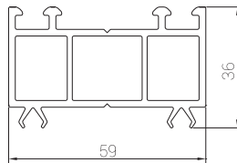
PR6037 Kasa Yükseltme Profili Frame Joint Profile
