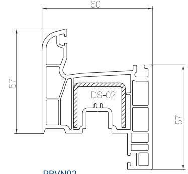
PRVN02 Kanat Profili Sash Profile
