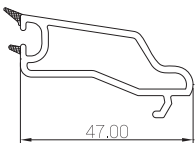
PR7114 Tek Cam Çıtası Single Glazing Bead
