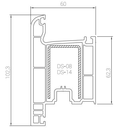
PRVN05 Dışa Açılım Kapı Profili Outside Opening Door Sash Profile
