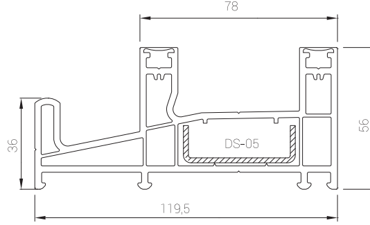
PRSY47 Sineklikli Kasa Profili Frame Fly Screen Profile
