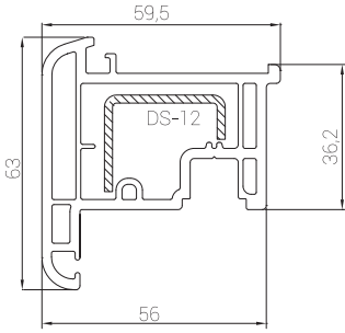
PRVN13 Hareketli Orta Kayıt Profili Overhang (Stump)
