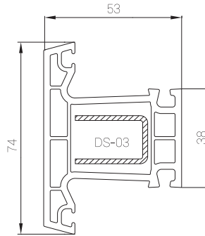
PRFS03 Orta Kayıt Profili Mullion Profile
