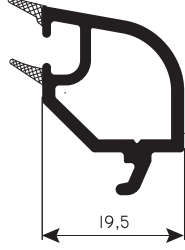
PRVN17 20mm Çift Cam Çıtası 20mm Double Glazing Bead
